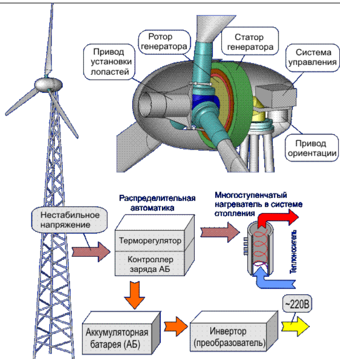
Рис. 1. Ветровая электростанция
